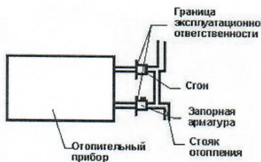
Рис.2 система отопления
