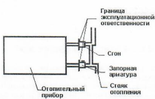
Рис.2 система отопления
