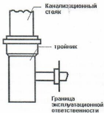
Рис.1 система водоотведения
