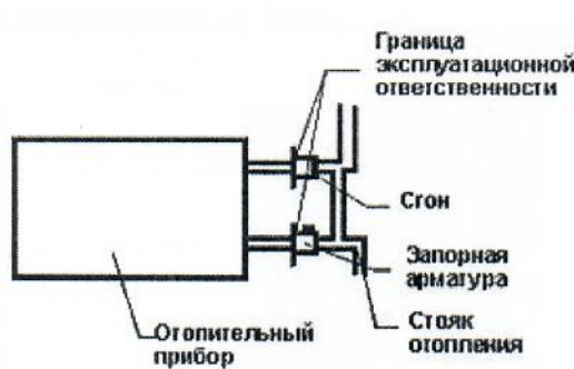
Рис.2 система отопления
