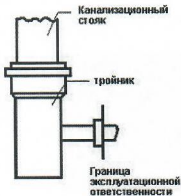
Рис.1 система водоотведения
