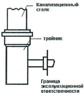
Рис.1 система водоотведения
