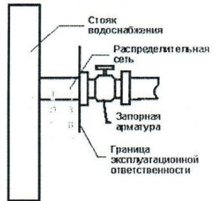
Рис.3 система водоснабжения
