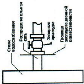
Рис.3 система водоснабжения
