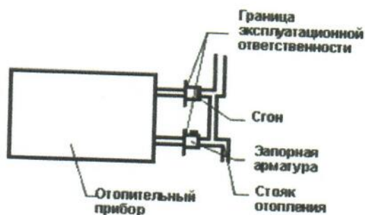
Рис.2 система отопления
