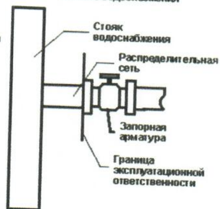
Рис.3 система водоснабжения
