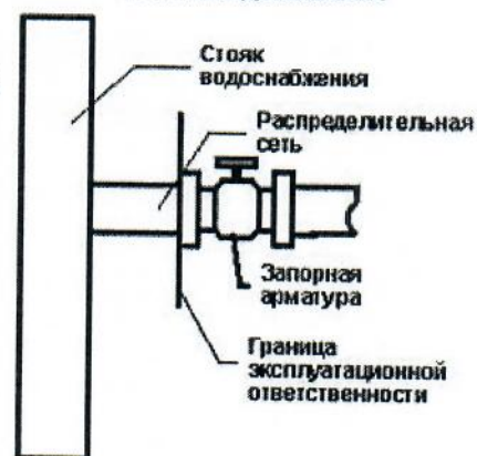
Рис.3 система водоснабжения
