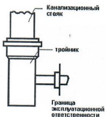
Рис.1 система водоотведения
