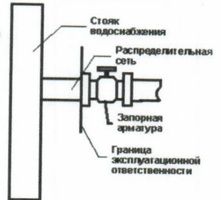
Рис.3 система водоснабжения
