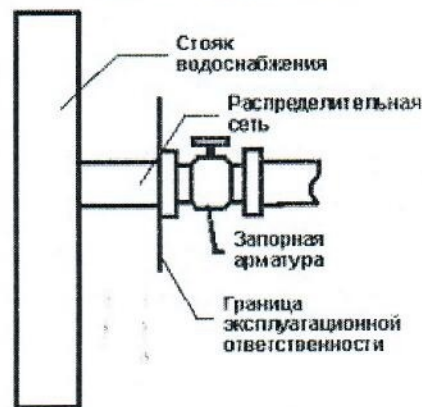
Рис. 3 система водоснабжения
