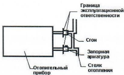
Рис.2 система отопления
