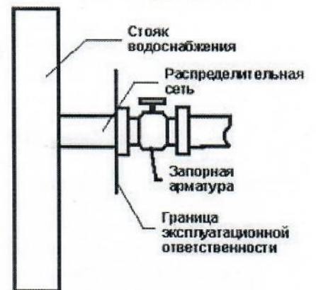
Рис.3 система водоснабжения
