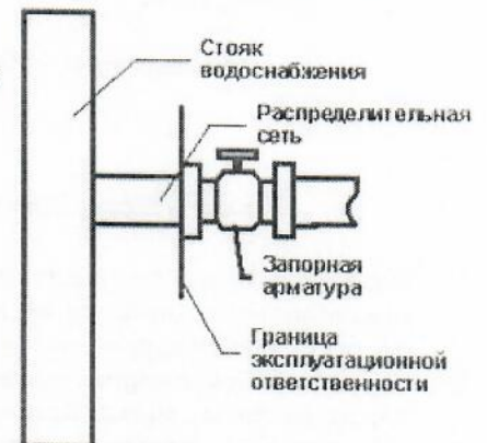
Рис.3 система водоснабжения
