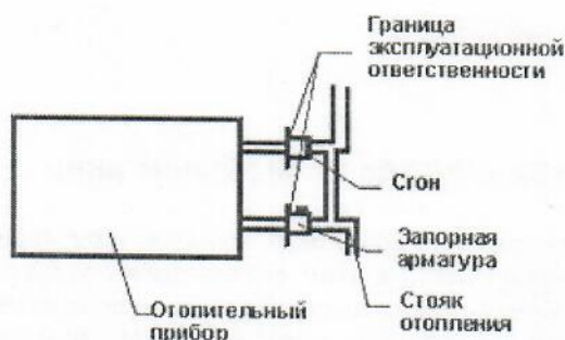
Рис.2 система отопления
